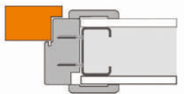
Монтаж в гипсокартонную стену с помощью болтов
