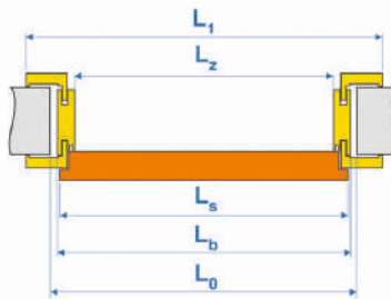
С КОРОБКой ECO-FIT
