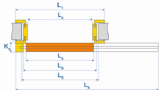
РАЗДВИЖНАЯ СИСТЕМА ECO-SLIDE С КОРОБКой ECO-FIT
