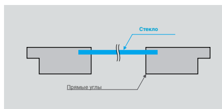
Стекло установлено с смещением под фальц полотна
