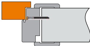
Монтаж в бетонную стену с помощью анкеров
