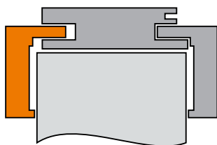
Сечение дверной коробки
