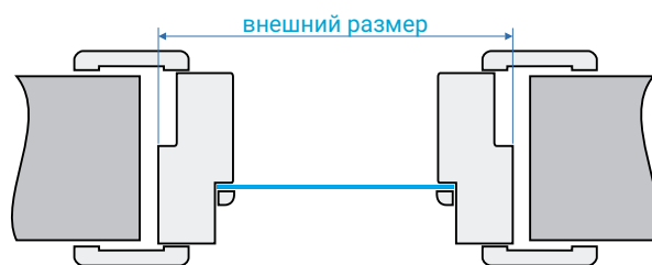
Конструкция фрамуги в исполнении STANDART
