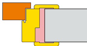
Монтаж в бетонную стену за допомогою монтажної піни
