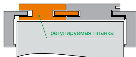
Сечение дверной коробки с регулирующей планкой и шпонкой
